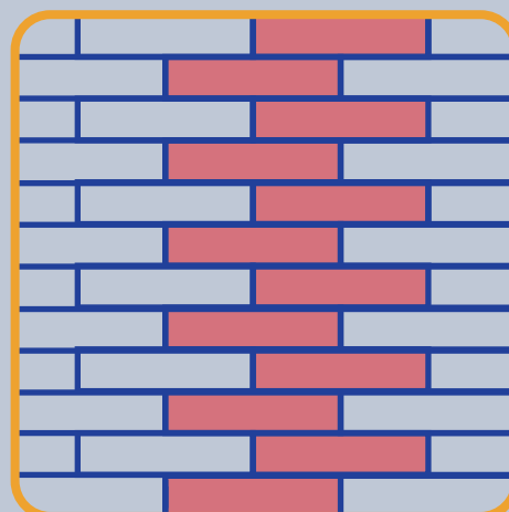
C. HALFSTEENSVERBAND
