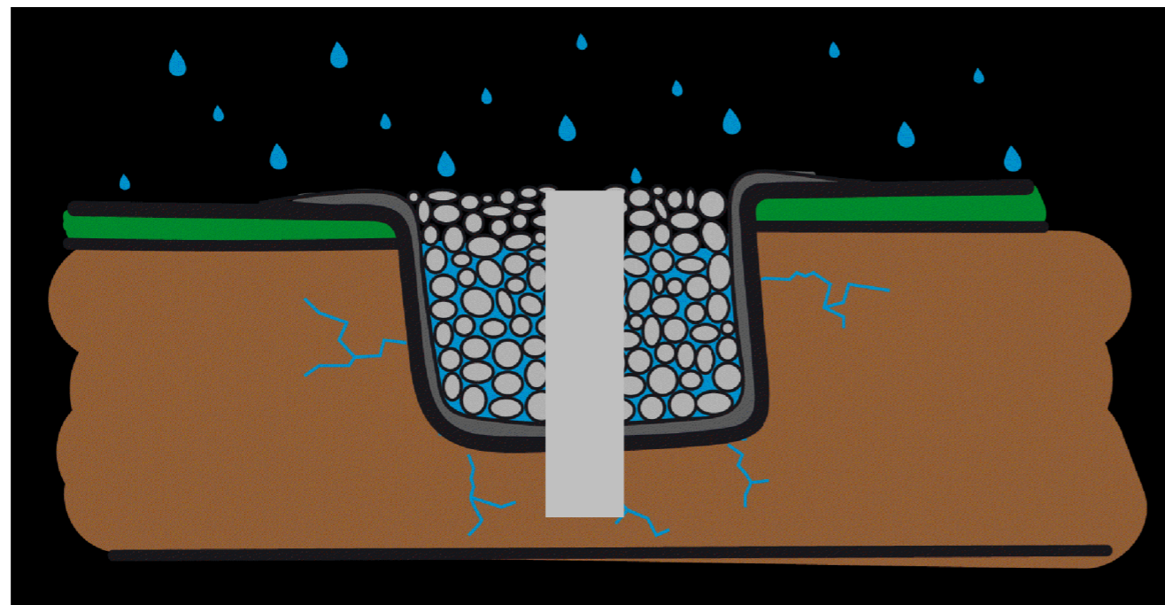
OIO-put voor ontluftung vuilwater in grindkoffer
