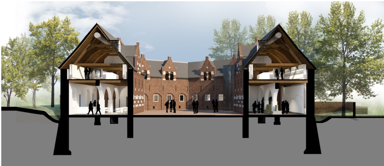
Doorsnede van het ontwerp van het Kruithuis
